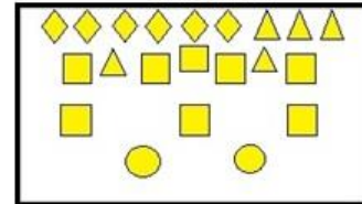
Хаотична
