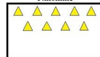
Симетрична
