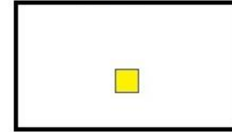
Симетрична
