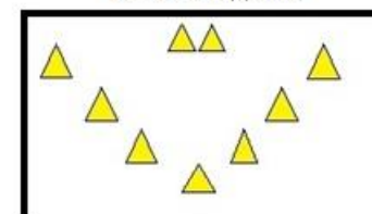
Клиноподібна
