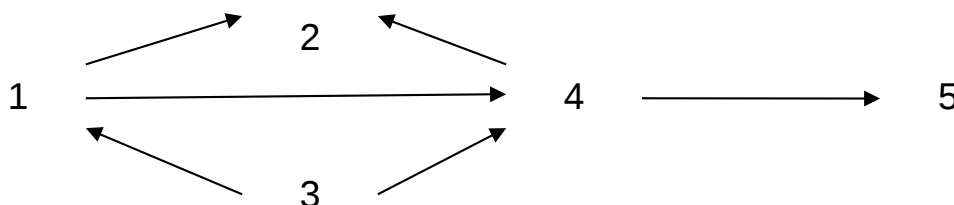
Рис. 6.1. Стрілчастий графік
